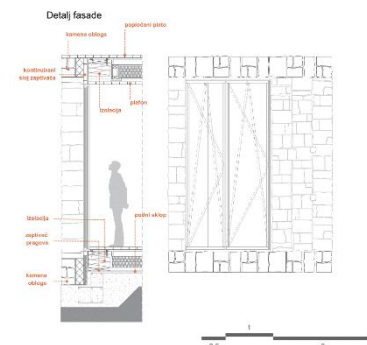
Slika 8. Detalj fasade
